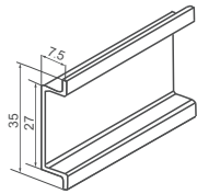
TH35-7.5 DIN Rail
