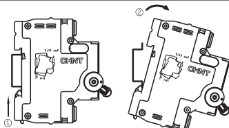
TH35-7.5 DIN Rail
