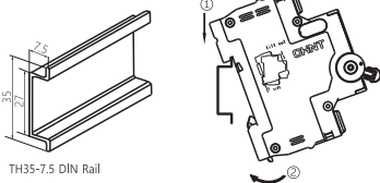
TH35-7.5 DIN Rail
